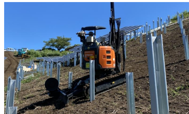
同社が自社開発した特殊重機による ダウンザホールハンマー工法
